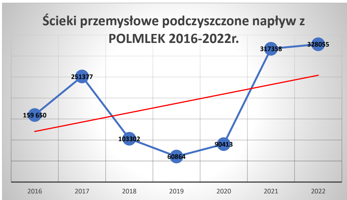
Wykres nr 10: Napływ ścieków przemysłowych z POLMLEK do oczyszczalni ścieków w latach 2016-2022 w tys m 3 .
