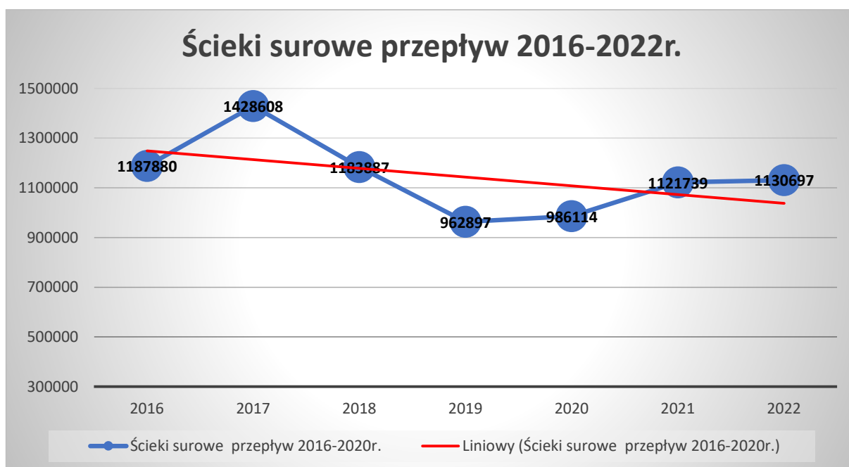
Wykres nr 9: Napływ ścieków surowych do oczyszczalni ścieków w latach 2016-2022 w mln m 3 .
