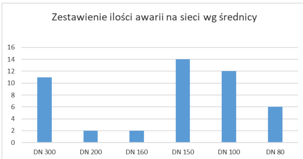
Wykres nr 3: Zestawienie ilości awarii na sieci wg średnic w 2022 r.
