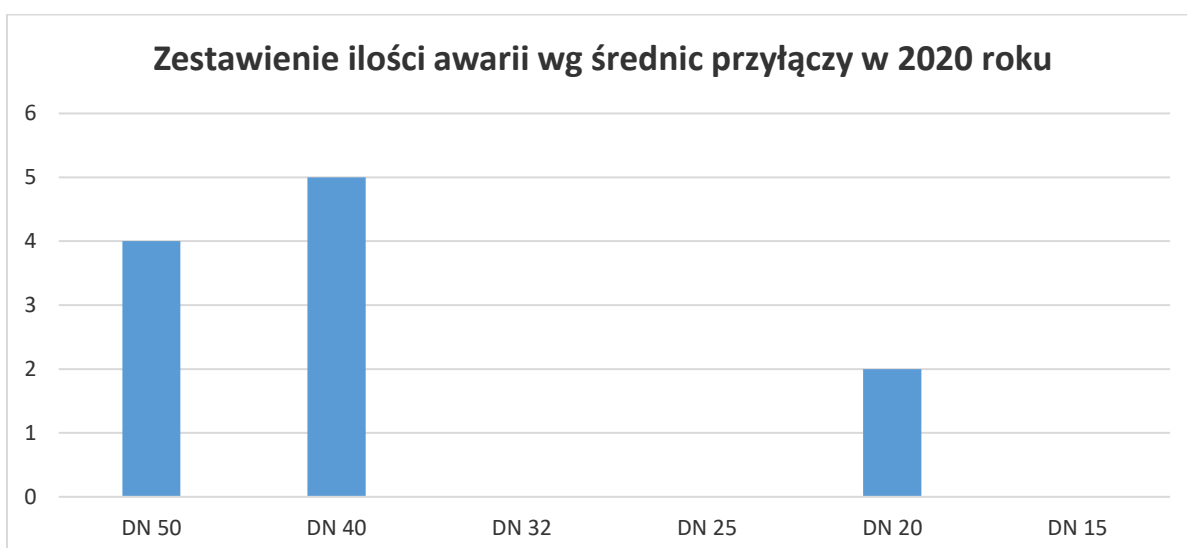
Wykres nr 4: Awarie wg średnic przyłączy w 2020 r.
