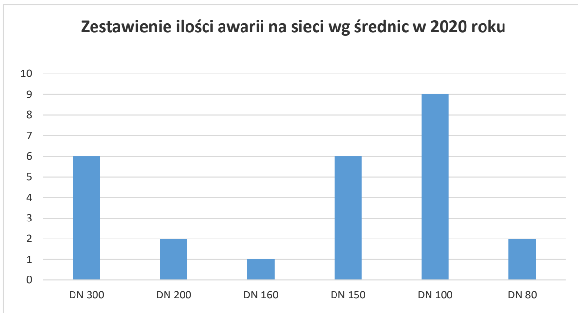
Wykres nr 3: Awarie na sieci wg średnic w 2020 r.
